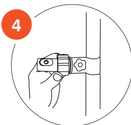
4 Visser le collier de serrage sur l'anneau de fixation
